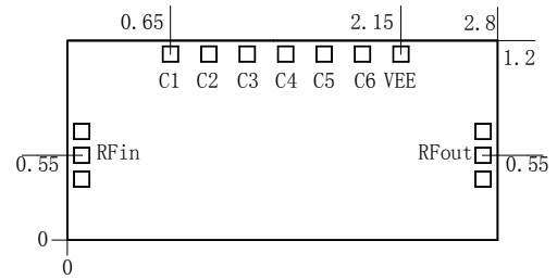
推荐装配图
