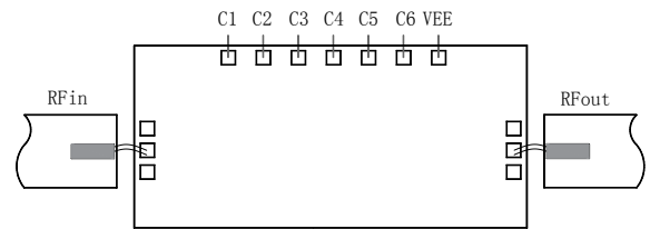
推荐装配图
